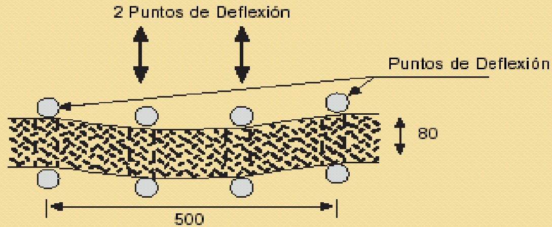
Fig. 2: Ensayo Dinámico de Deflexión de 4 Puntos a 0,4 MPa
